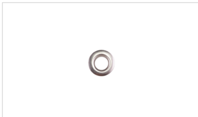
REFERENCIA: I-50B Ilhós DESCRIPCIÓN: I - 50B Ilhós MATERIAL: Hierro o Latón
