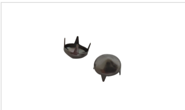
REFERENCIA: Cravo 9,0 Cone DESCRIPCIÓN: Clavel 9,0 Cone MATERIAL: Grafite DIMENSIONES: 9mm (cabeza)
