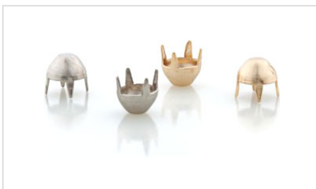
REFERENCIA: Cravo 7,0 Ponta Chata DESCRIPCIÓN: Clavel 7,0 Ponta Chata MATERIAL: Latón DIMENSIONES: 7mm (cabeza)
