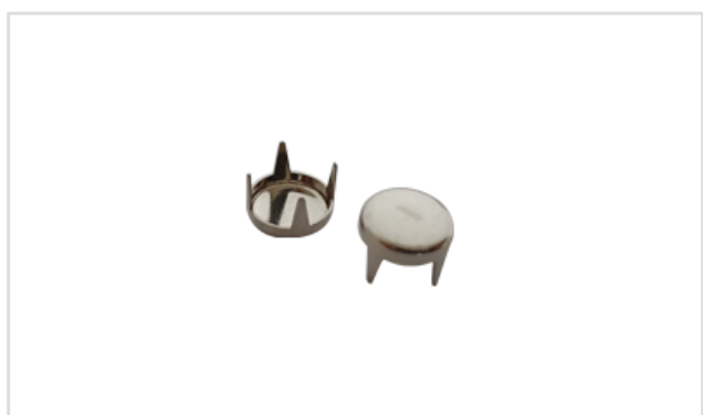
REFERENCIA: Cravo 7,0 Chato 7-45 DESCRIPCIÓN: Cravo 7,0 Chato 7-45 MATERIAL: Hierro o Latón DIMENSIONES: 7,0mm (cabeza)
