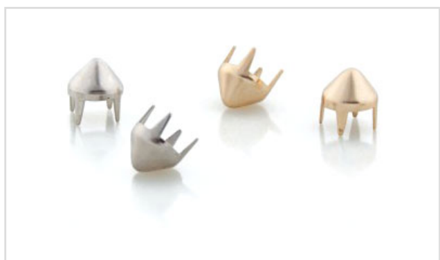
REFERENCIA: Cravo 7,0 Ponta (SPIKE) DESCRIPCIÓN: Clavel 7,0 Ponta (SPIKE) MATERIAL: Hierro o Latón DIMENSIONES: 7mm (cabeza)
