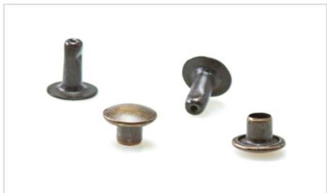
REFERENCIA: Rebite 1,0 PE 6,0mm DESCRIPCIÓN: Remache 1,0 PE 6,0mm MATERIAL: Hierro o Latón DIMENSIONES: 7mm (cabeza) 6mm (altura)
